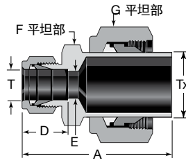
1 in. 以上
